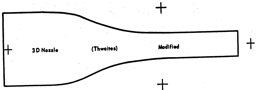
Fig. 5—Nozzle Profile
