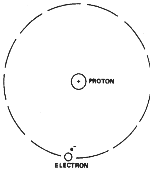
Figure 7. Actual hydrogen atom.
